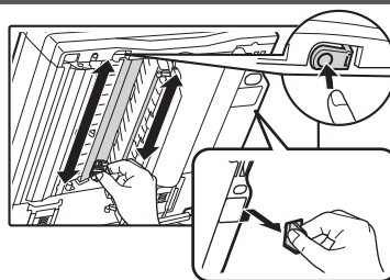
Papierinvoerrol
