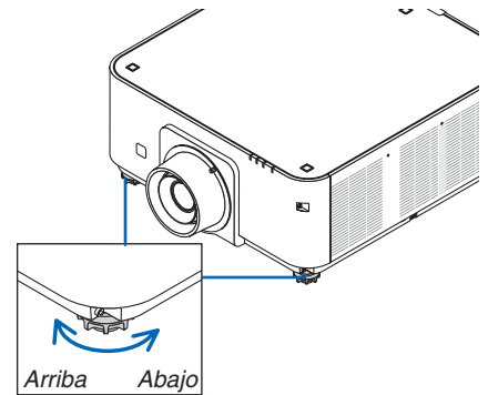
Pata de inclinación (hay una más en la parte trasera)
