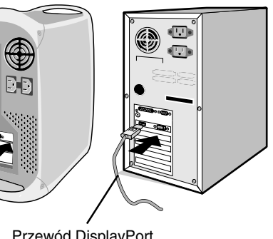
Przewód DisplayPort (brak w zestawie) Rysunek B.2
