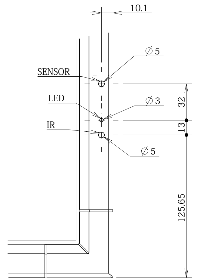
section A scsle 1:2
