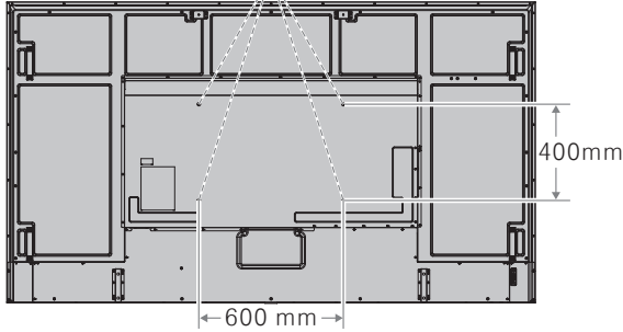
마운트 인터페이스(M8)
